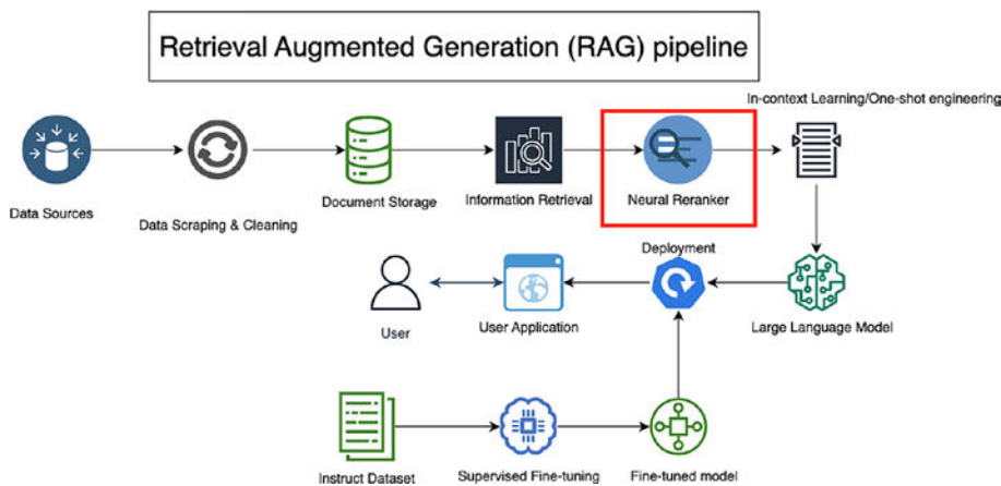
Figure 9-7. RAG reranker
